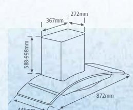
MDH-922OC
