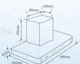
MDH-936STHC
